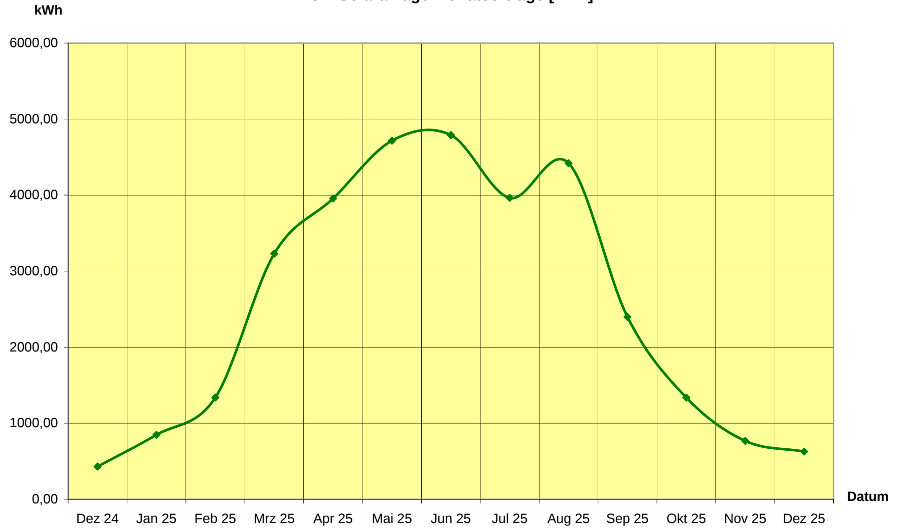
BSM Solaranlage Monatserträge [kWh]
